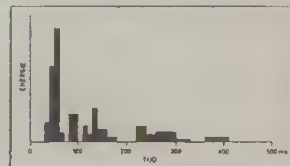
fig. 7 Voorbeeld van het energieverloop in een concertzaal na aankomst van het directe geluid op tijd t = 0 (naar Kronstad)
